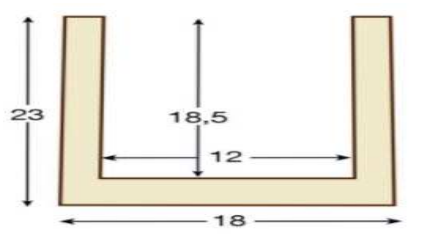
VIGA 318
